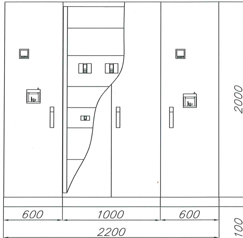
Внешний вид, двери. Фальшпанели защитные распределительной панели
