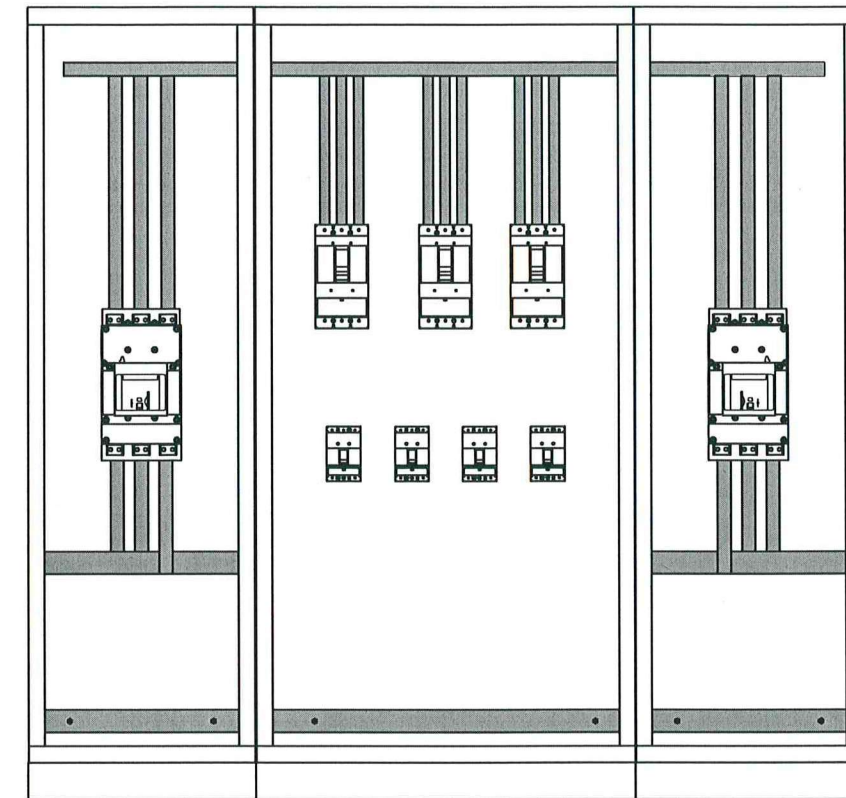
Внешний вид без дверей и Фальшпанелей
