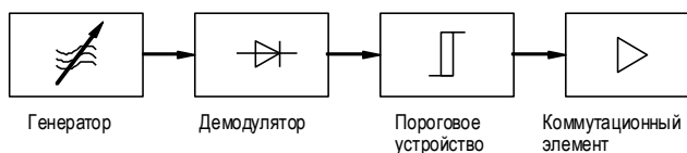
Рис. 2 - Функциональная схема выключателей.
