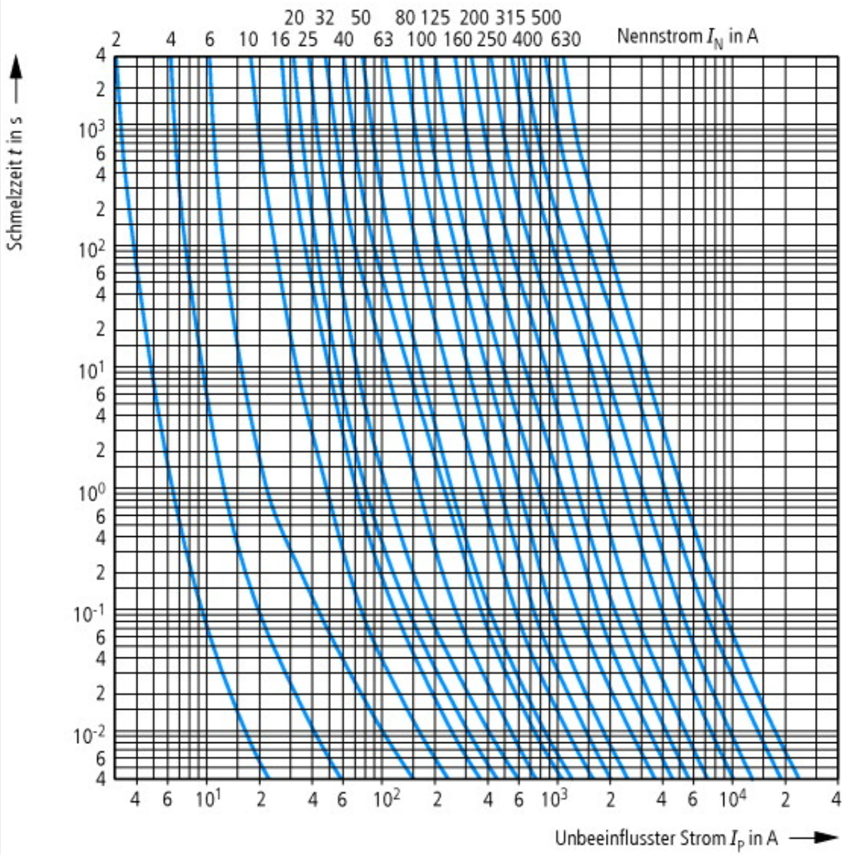
Zeit-Stromkennlinie
